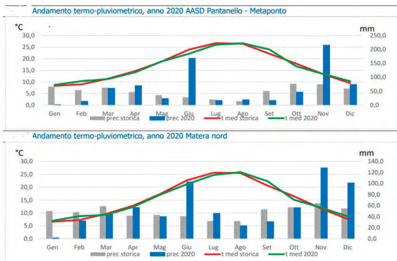
Figura 21. Andamento termo-pluviometrico in Basilicata anno 2020
